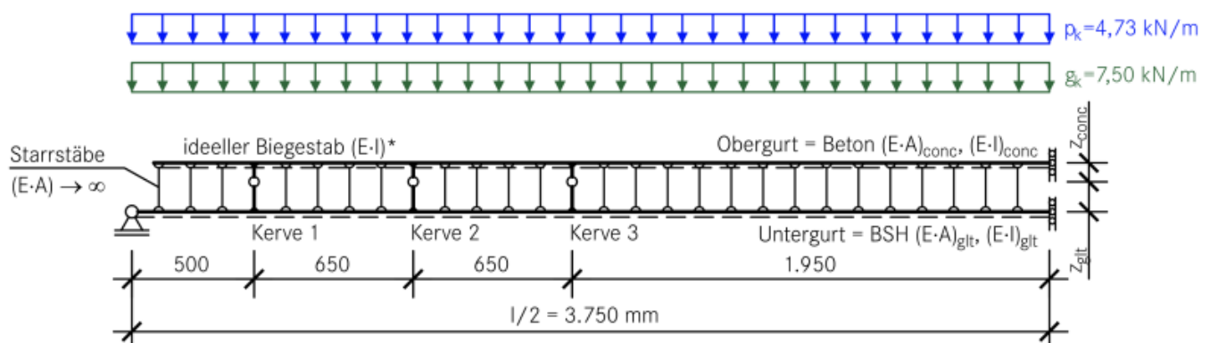
Abb. 3: Stabwerkmodell nach Rautenstrauch mit Einwirkung
